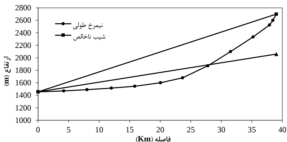
شکل ۴. نمایش نیمرخ طولی، شیب ناخالص و شیب خالص در طول مسیر رودخانه گیان
