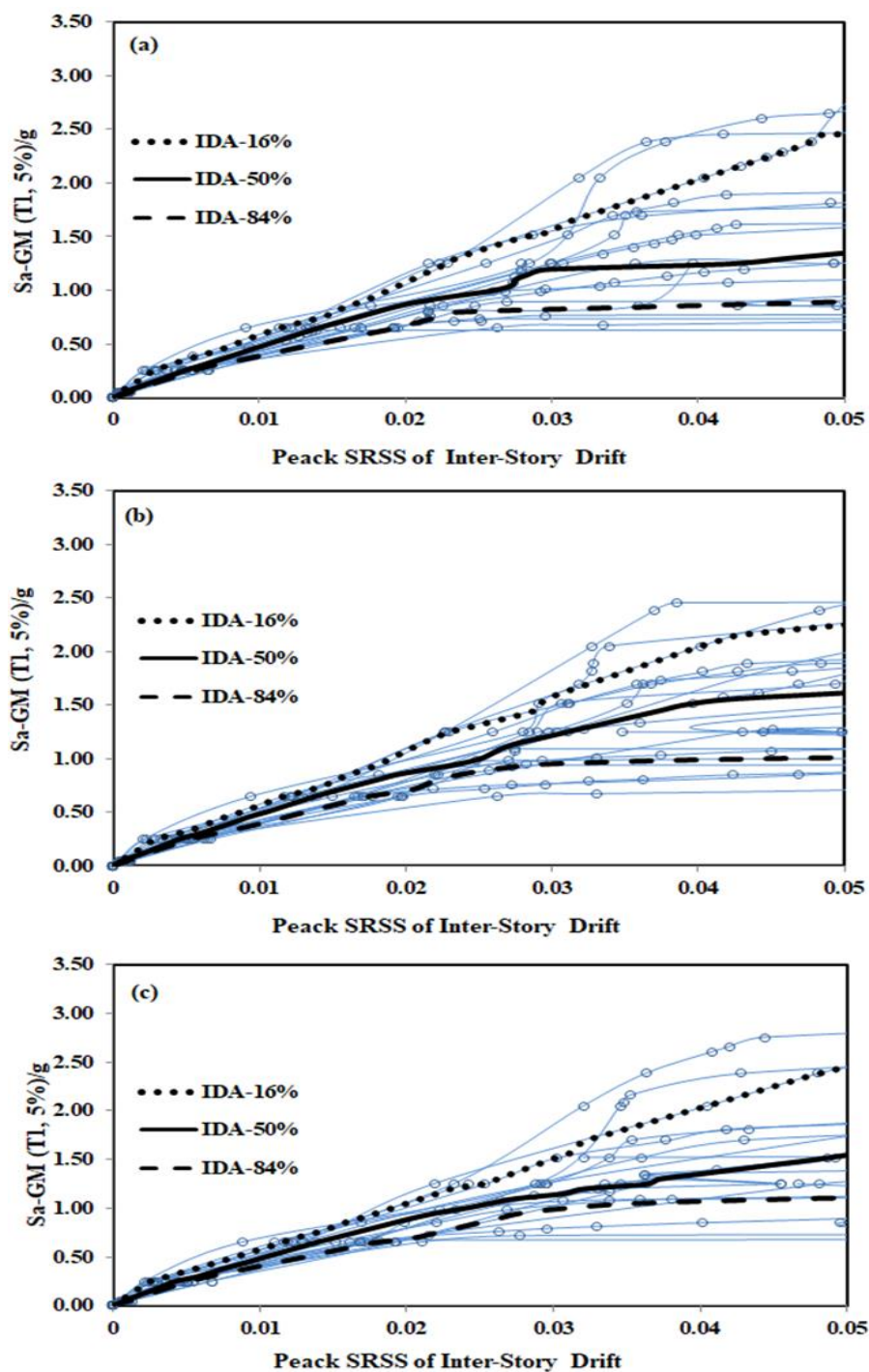
شکل ۸. نمودارهای IDA ساختمان نه طبقه با خروج از مرکزیت e_d/A=9\% . (a) مدل آئین‌نامه‌ای؛ (b) مدل بالانس-۲۵٪؛ و (c) مدل متقارن مقاومتی
