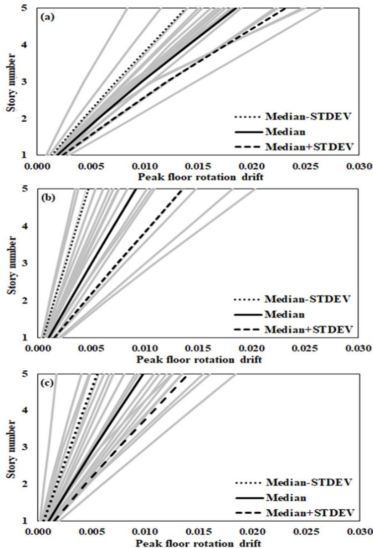
شکل ۱۲. نمودار حداکثر دریافت چرخش سقف‌های ساختمان پنج طبقه در طبقات مختلف و در سطح شتاب طیفی فروریزش با e_d/A=12\% : (a) مدل آئین‌نامه‌ای؛ (b) مدل بالانس-۲۵٪؛ (c) مدل متقارن مقاومتی
