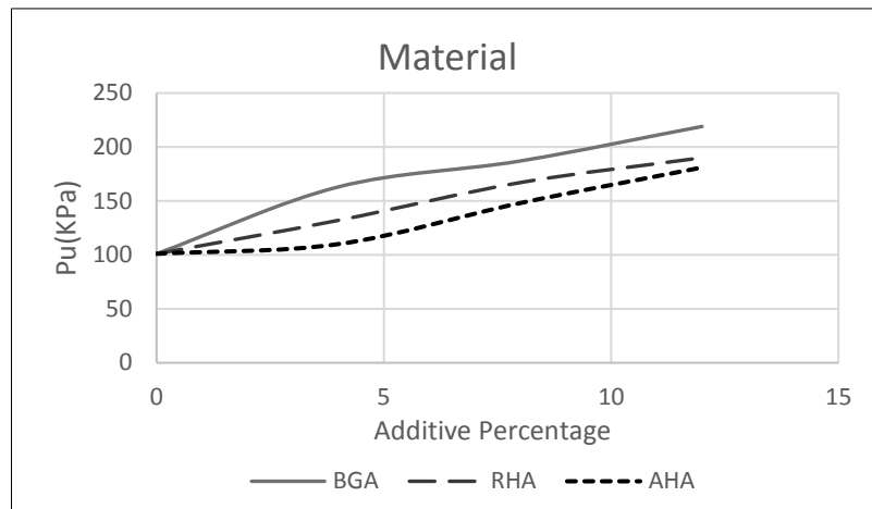
شکل ۵. نمودار مقاومت تک محوری بر حسب درصد افزودنی
