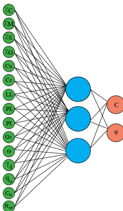
شکل ۴. نمایی از ورودی‌ها و خروجی‌های شبکه عصبی Fig. 4. Input and output of neural network
