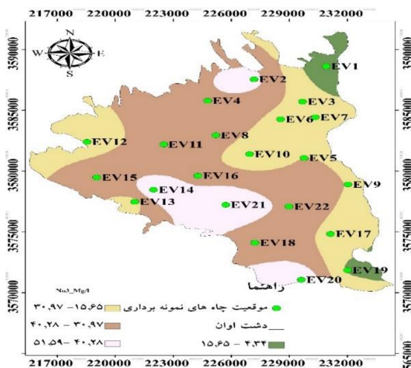
شکل ۵. نقشه توزیع مکانی یون نیترات در آب زیرزمینی آبخوان اوان
