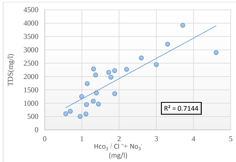
شکل ۷. نمودار نسبت یونی ( \text{HCO}_3^-/\text{Cl}^-+\text{NO}_3^- ) در مقابل (TDS)
