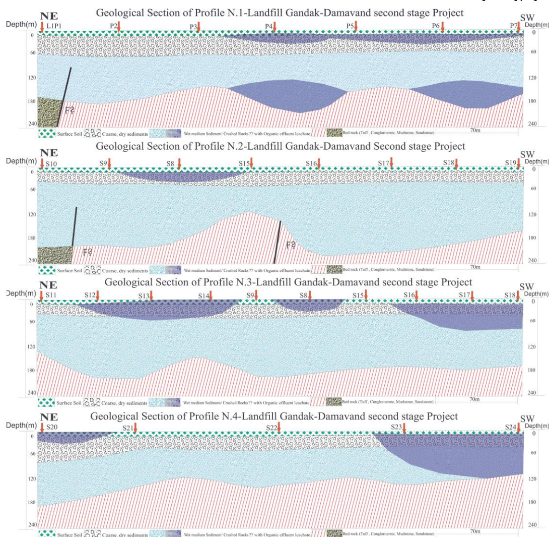
شکل ۱۰. مقطع زمین‌شناسی در امتداد پروفیل اول تا چهارم
