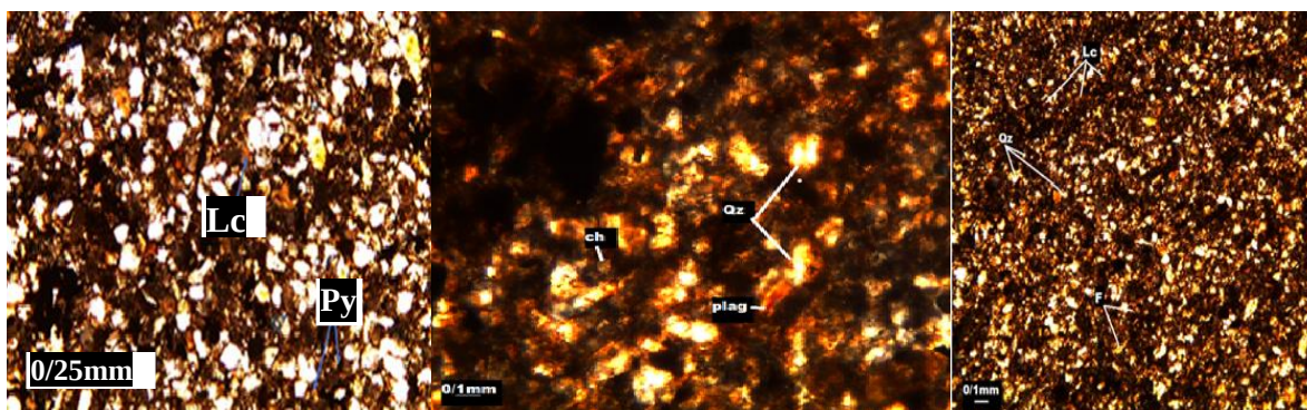
شکل ۵. تصاویر میکروسکوپی نمونه ماسه‌سنگ: Qz: کوارتز، Mus: مسکویت، F: فلدسپات پلاژیوکلاز، Slm: اسلیت و فیلیت،
