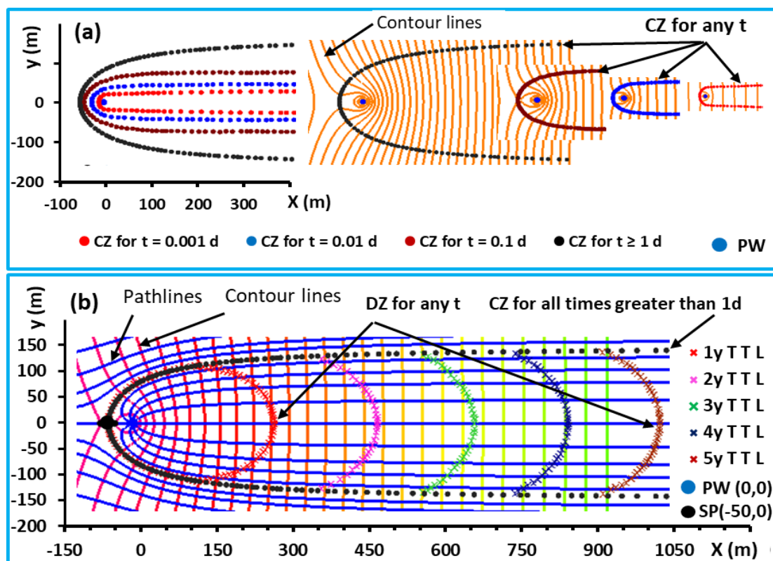
شکل ۱۱. اثر تداوم پمپاژ (t): (a) چگونگی گسترش حریم آبریز. (b) چگونگی گسترش حریم تخلیه. خطوط زمان گذر یک ساله هستند.
