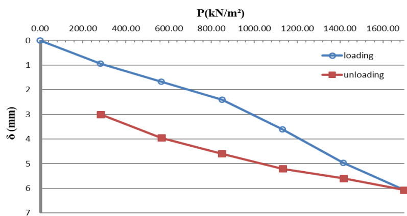
شکل ۴- نتایج آزمایش بارگذاری صفحه اول
