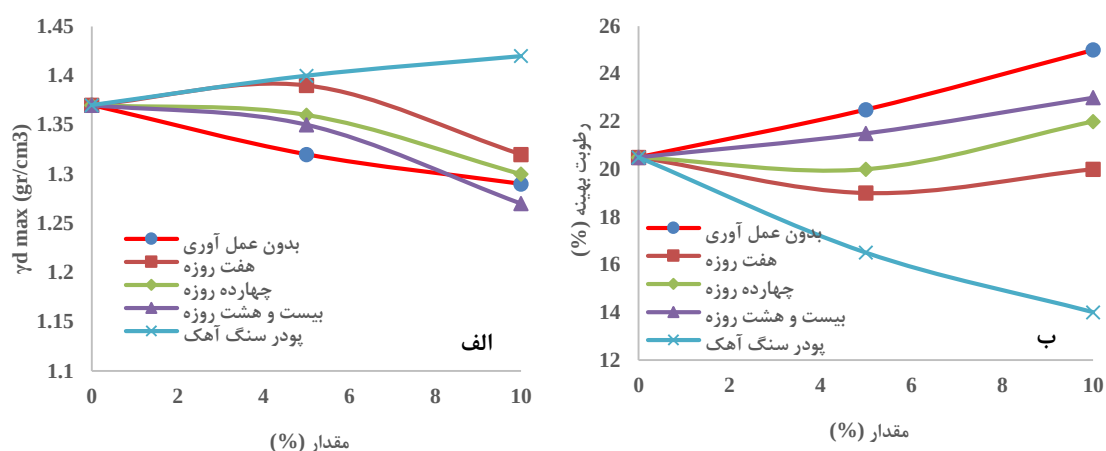
شکل ۴: تأثیر نانو رس و پودر سنگ آهک بر روی نتایج آزمون تراکم خاک رس مورد مطالعه، الف- وزن مخصوص خشک حداکثر، ب- رطوبت بهینه.
