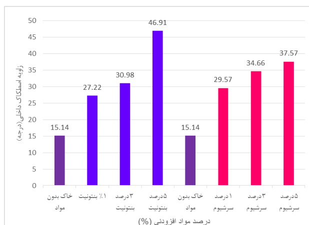
شکل ۸. نمودار تأثیر درصد‌های وزنی مختلف بنتونیت و سریشم بر روی زاویه اصطکاک داخلی خاک رسی
