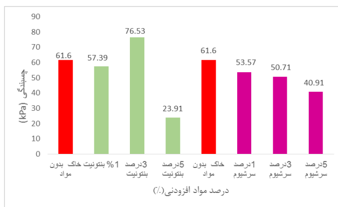
شکل ۷. تأثیر درصد‌های وزنی مختلف بنتونیت و سریشم بر روی چسبندگی خاک رسی
