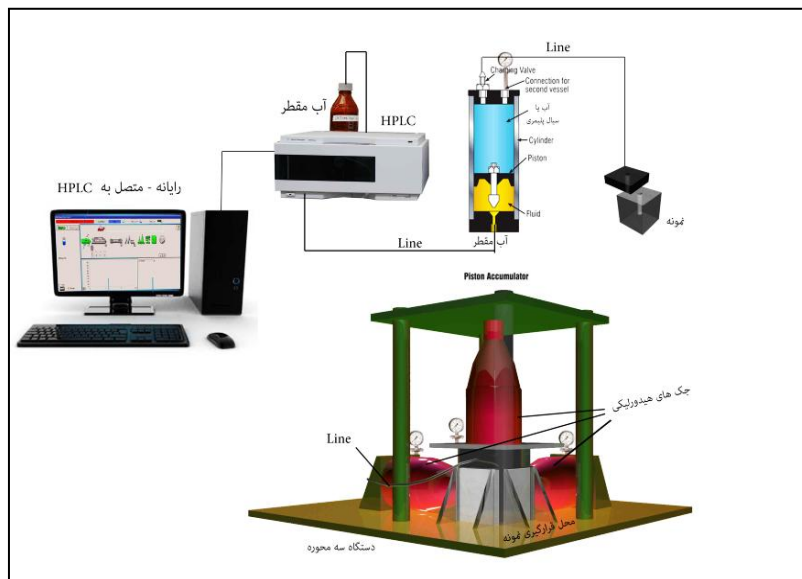
شکل ۶. تجهیزات آزمایشگاهی و نحوه اعمال تنش های برجا
