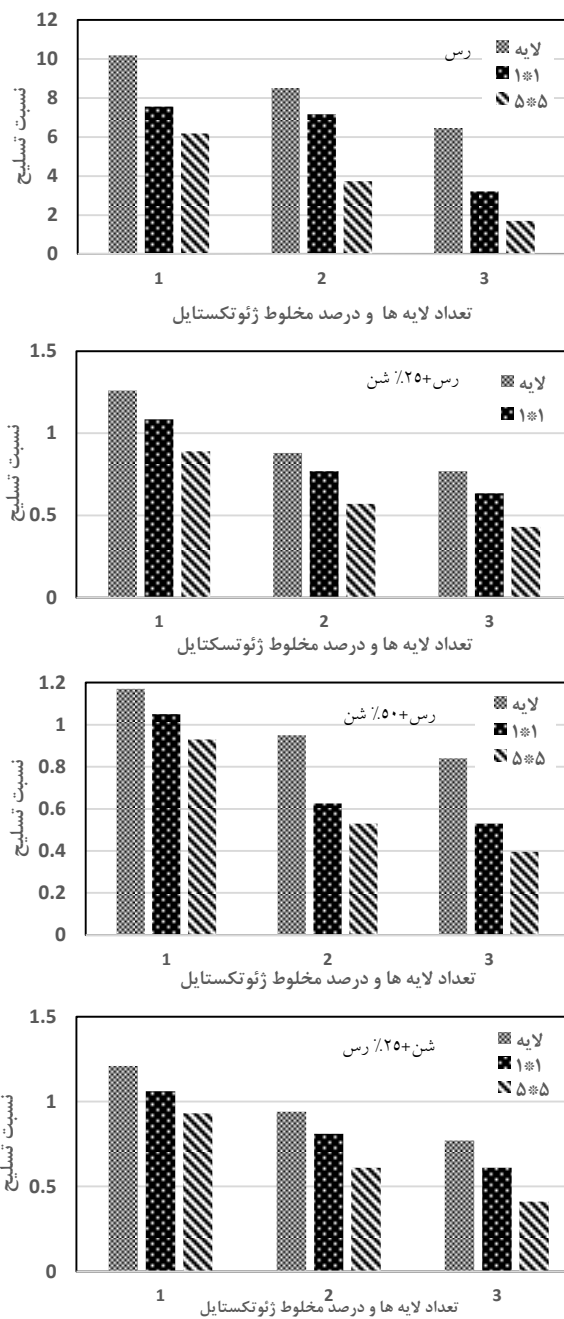
شکل ۲۰. تأثیر نحوه کاربرد ژئوتکستایل در نسبت تسلیج نمونه‌های بررسی شده (حالت خشک)
