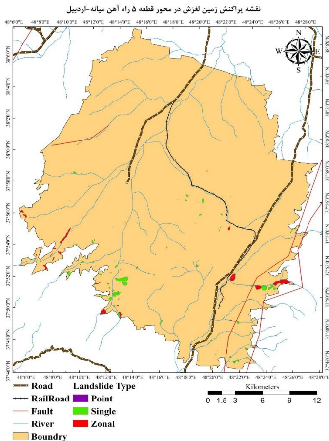
شکل ۳. نقشه پراکنش زمین لغزش‌های نقطه‌ای، منفرد و پهنه‌ای رخ داده در قطعه ۵ راه آهن اردبیل-میانه
