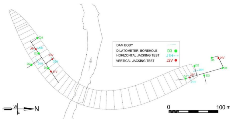
گالری‌های LG1 و RG3 ساختگاه سد بهشت آباد [۳۴]
