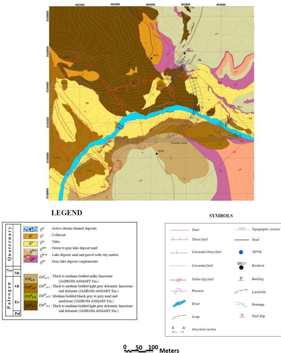
شکل ۱. پلان زمین‌شناسی ساختگاه سد بهشت‌آباد [۳۴]
