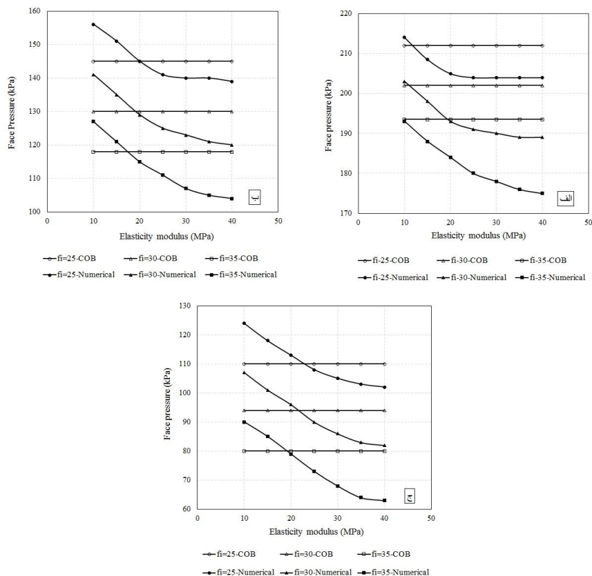
شکل ۷. مدول الاستیسیتة- فشار جبهه کار برای تراز آب الف (۰، ب ۹، ج ۲۷ متری از سطح زمین)
