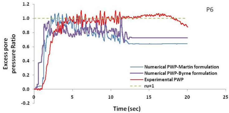
شکل ۱۲. مقایسه تاریخچه نسبت فشار آب حفره‌ای مدل‌سازی عددی و آزمایش ساتریفور در عمق ۲/۶ متر
