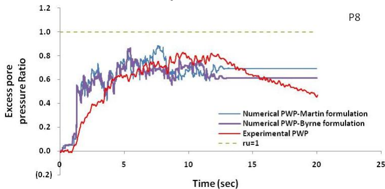
شکل ۱۴. مقایسه تاریخچه نسبت فشار آب حفره‌ای مدل‌سازی عددی و آزمایش ساتریفور در عمق ۷/۵ متر
