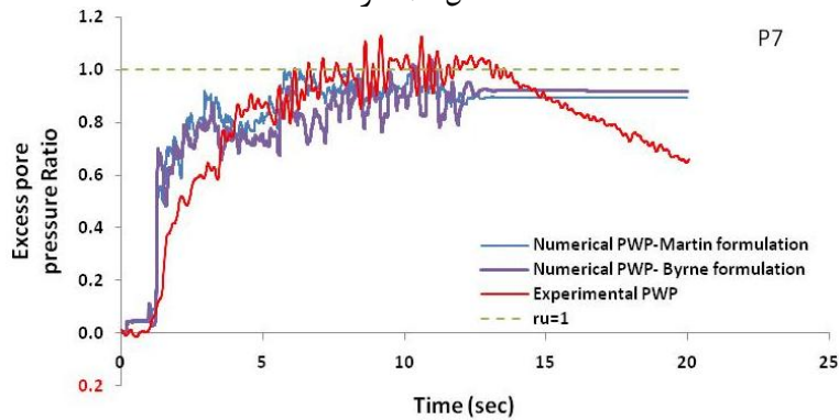
شکل ۱۳. مقایسه تاریخچه نسبت فشار آب حفره‌ای مدل‌سازی عددی و آزمایش ساتریفور در عمق ۵ متر
