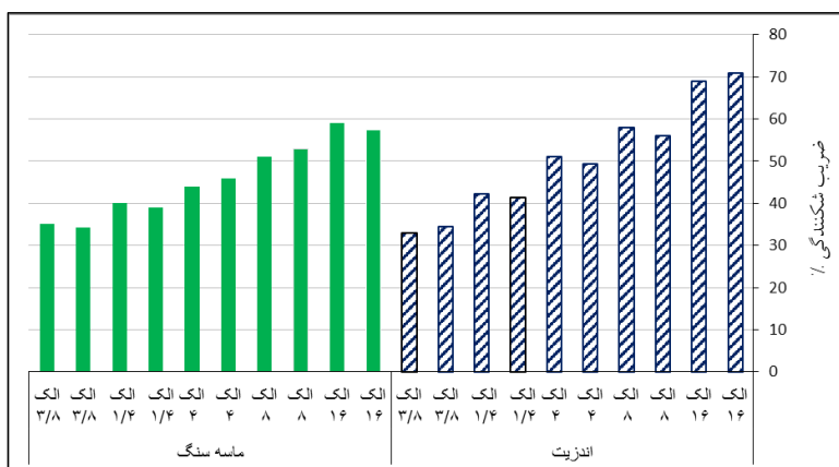
شکل ۱۱. نمودار ضرایب ساینده و شکندگی در برابر سایز دانه‌ها در دو جنس غالب مسیر (آندزیت و ماسه‌سنگ)
