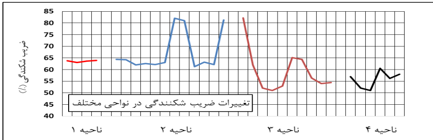
شکل ۸. نتایج ضریب قابلیت شکنندگی برای هر یک از آبرفت‌های نواحی ۴ گانه مسیر تونل خط دو مترو تبریز
