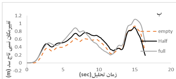
شکل ۹. تغییر مکان نسبی تاج سد در سه حالت خالی، نیمه پر و پر برای زلزله‌های الف) طبس و ب) سانفرانسیسکو
