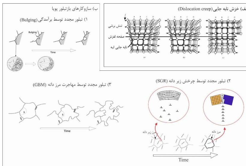
شکل ۲. سازوکارهای دگرشکلی در مقیاس میکروسکوپی، (الف) خزش ناب‌جایی، (ب) سازوکارهای باز تبلور پویا
