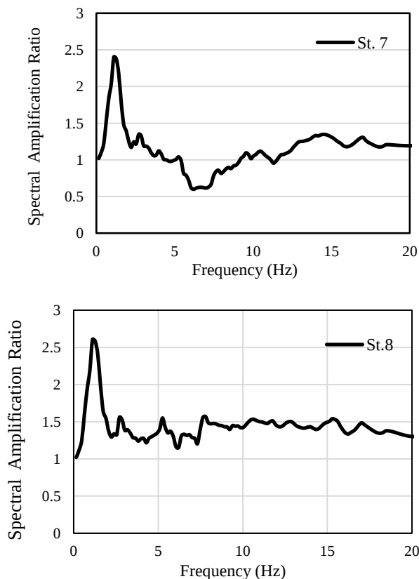
شکل ۵. توابع تقویت طیفی در ایستگاه‌های مختلف واقع بر یال دره
