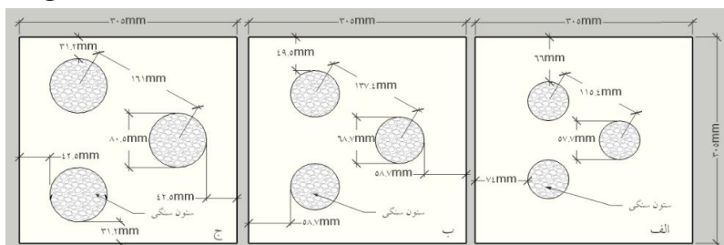
شکل ۵. آرایش قرارگیری ستون‌های سنگی در آرایش مربعی الف (ب/۸/۴، ب/۱۲/۴، ج/۱۶/۴)
