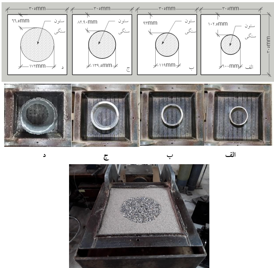
شکل ۴. آرایش قرارگیری ستون‌های سنگی منفرد الف) ۸/۴؛ ب) ۱۲/۴؛ ج) ۱۶/۴؛ د) ۲۵/۴
