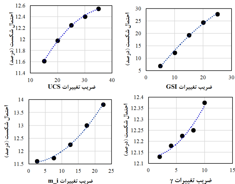
شکل ۱۵. تجزیه حساسیت احتمال شکست سازه شیروانی جناح راست سرریز برای حالت بعد از باربرداری برحسب ضریب تغییرات کمیت‌ها
