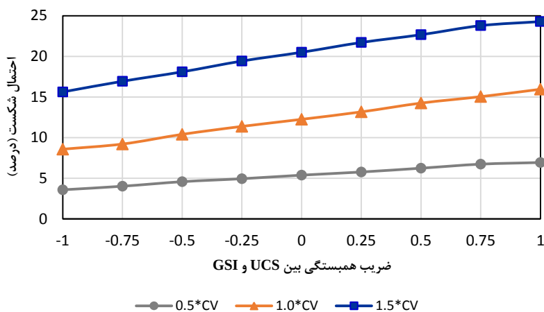
شکل ۱۹. تأثیر ضریب همبستگی بین مقاومت فشاری تک محوری و شاخص مقاومت زمین شناسی بر احتمال شکست شبه استاتیکی شیریانی جناح راست سرریز برای حالت بعد از باربرداری
