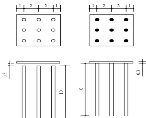
شکل ۵. نمای پلان و کنار ابعاد و محل اتصال پی رادیه-شمع متصل (سمت راست) و منفصل (سمت چپ) (واحد: متر)
