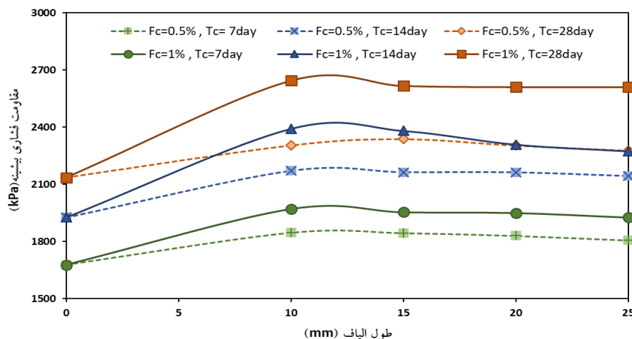
شکل ۲. تغییرات مقاومت فشاری بیشینه خاک-سیمان با ۸ درصد سیمان ( C_c = 8\% ) و مسلح شده با ۰/۵ و ۱ درصد الیاف (۰/۱٪ و ۰/۵٪) در طول‌های مختلف و زمان‌های عمل‌آوری ( T_c = 7, 14, 28 روزه) (۷، ۱۴، ۲۸ روزه)
