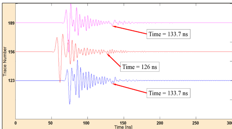
شکل ۸. سه تریس انتخابی از نگاشت راداری در موقعیت ۹/۸۴ (تریس ۱۲۳)، ۱۲/۴۸ (تریس ۱۵۶) و ۱۵/۱۲ متری (تریس ۱۸۹) طول مدل ۲۳
