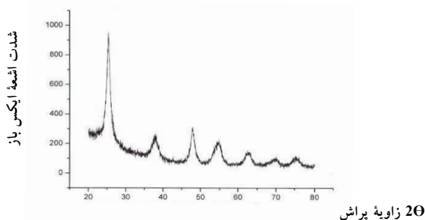
شکل ۵. پراش XRD نمونه نانو مواد کربنات کلسیم تصویر میکروسکوپ الکترونی روبشی از نانوکربنات کلسیم استفاده شده در طرح در شکل ۶ مشاهده می‌شود.
