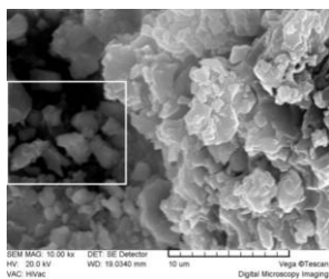
شکل ۵. تصاویر SEM تهیه شده از نمونه بهسازی شده به روش بیولوژیکی
