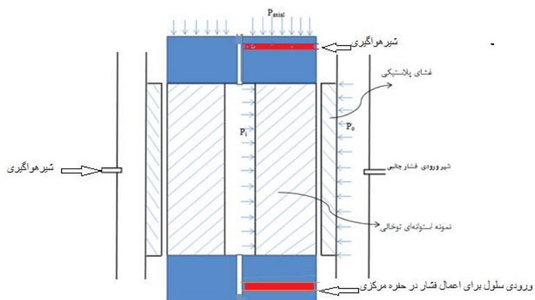
شکل ۳. نمایی از طراحی انجام شده برای اعمال فشار داخلی در سلول هوک تغییر یافته (در شکل نشان‌دهنده تنش محوری، P_{axial} نشان‌دهنده تنش جانبی و P_0 نشان‌دهنده فشار در حفره مرکزی P_i نشان‌دهنده فشار در حفره مرکزی است)
