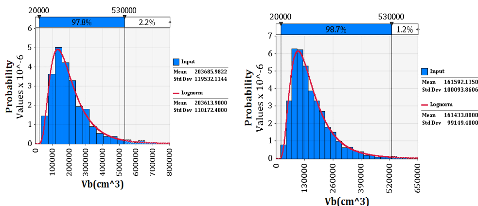
شکل ۵. توزیع حجم بلوک‌ها با فرض وجود درزه‌های غیرمداوم
