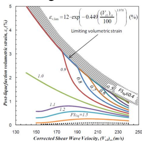
شکل ۱۳. نمودار ارتباط بین کرنش حجمی در لایه خاکی پس از روان‌گرایی با سرعت موج برشی اصلاح شده معادل ماسه تمیز (بی-۲۰۰۹) [۱۵]
