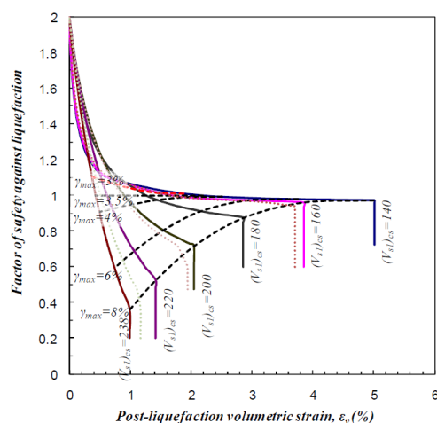
شکل ۱۲. نمودار ارتباط بین ضریب اطمینان در مقابل روان‌گرایی با کرنش حجمی در لایه خاکی پس از روان‌گرایی با توجه به سرعت موج برشی (بی-۲۰۰۹) [۱۵]
