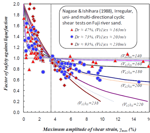
شکل ۱۱. نمودار اتباط بین حداکثر کرنش برشی ( \gamma_{max} ) و ضریب اطمینان در مقابل روان‌گرایی با توجه به سرعت موج برشی (بی-۲۰۰۹) [۱۵]
