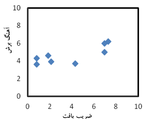
شکل ۳. ارتباط بین ضریب بافت و آهنگ برش
