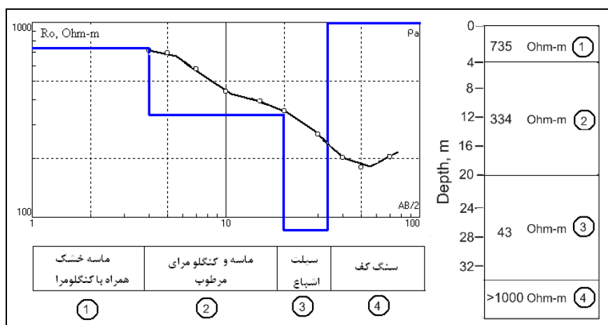
۵. نمودار چاهک الکتریکی و مدل ژئوالکتریکی مقطع زمین‌شناسی در محل پایه شرقی پل
