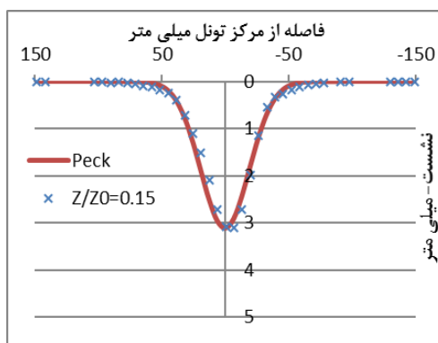
شکل ۷. نشست‌های ثبت شده و منحنی پک برازش شده برای چهار عمق مختلف برای ماسه متراکم
