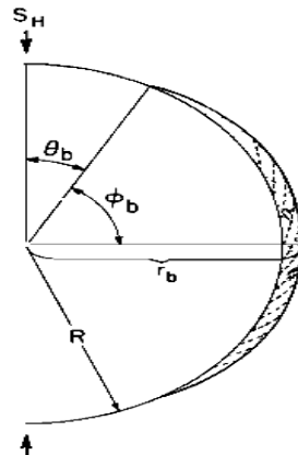
شکل ۲. عرض ( \phi_b ) و عمق شکستگی برشی ( r_b ) و مقدار زاویه با S_H ( \theta_b ) [۲۱].
