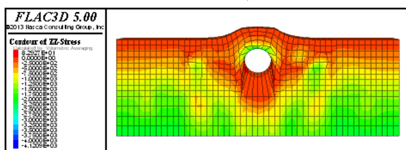
شکل ۸. کانتور تنش‌های قائم، پس از اعمال ۲۰۰ نیوتن نیروی برخاست لوله
