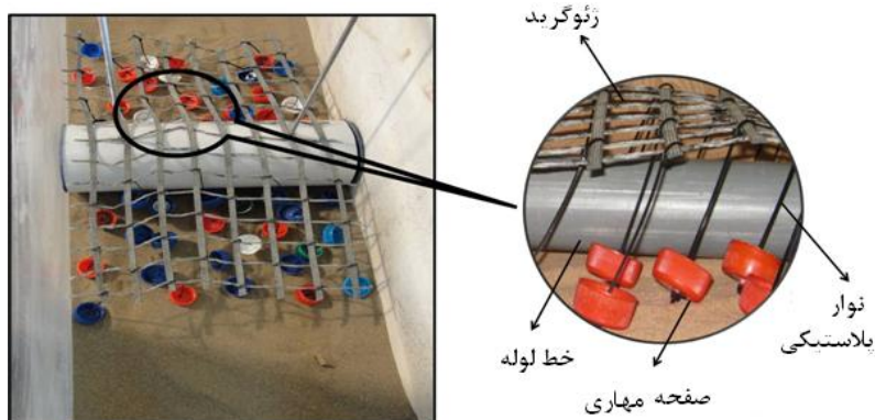
شکل ۲. استفاده از سیستم مهار- شبکه در آزمایشگاه
