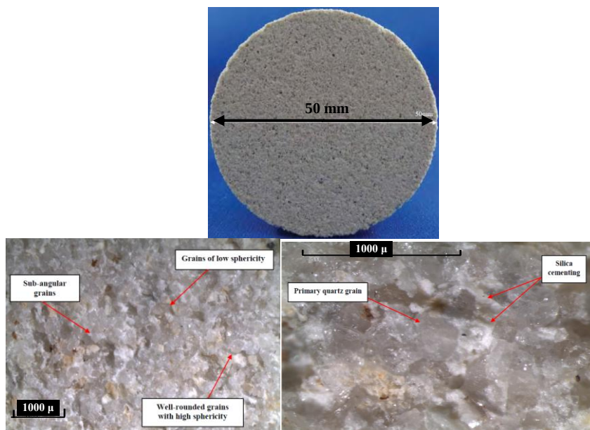
شکل ۳. الف) مقطعی از نمونه تهیه شده به قطر ۵۰ میلی‌متر، ب) نمایش توزیع و شکل دانه‌های اولیه کوارتز با مقیاس ۱۰۰۰ میکرون و ج) سیمان‌شدگی سیلیکاته دانه‌های اولیه با مقیاس ۱۰۰۰ میکرون
