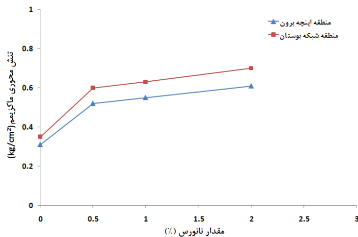
شکل ۱۴. تأثیر نوع خاک بر مقاومت فشاری محوری ماکزیمم نمونه‌ها ناشی از افزودن نانورس
