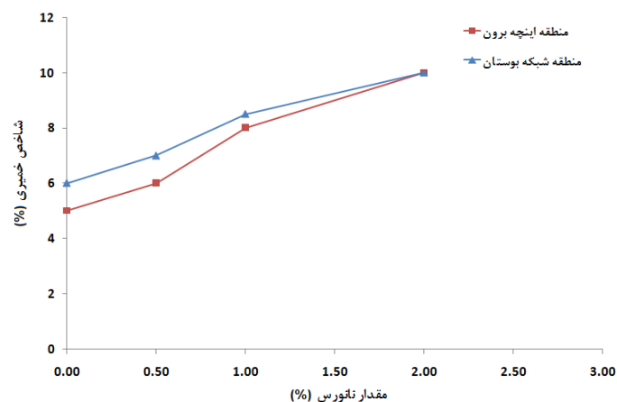
شکل ۱۳. تأثیر نوع خاک بر شاخص خمیری نمونه‌ها ناشی از افزودن نانورس
