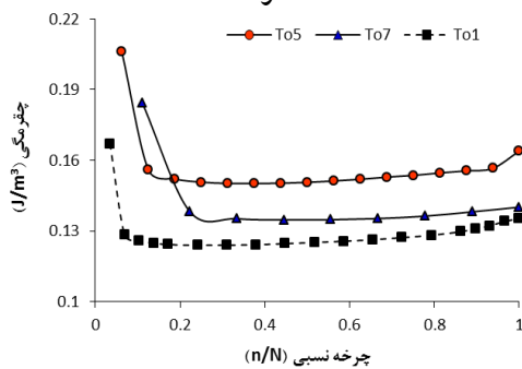
شکل ۹. روند تغییرات چگرمی و تغییرات انرژی وارفتگی در شرایط با بیشینه بار متفاوت
