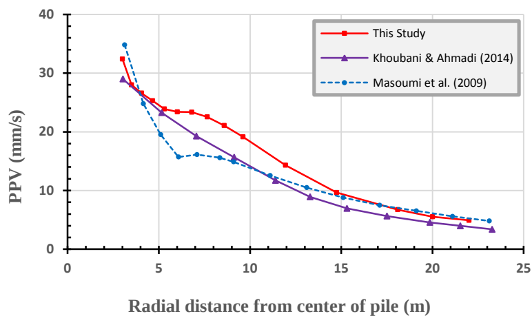
شکل ۱۱. مقایسه PPV برای ذرات سطح زمین برای شمع‌کوبی در لحظه قرارگیری نوک شمع در عمق ۵ متری با نتایج معصومی و همکاران (۲۰۰۹) و خوبانی و احمدی (۲۰۱۴)
