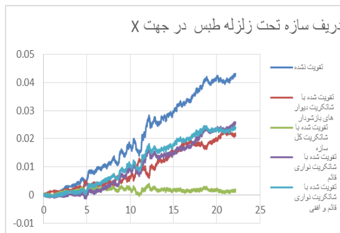
شکل ۱۲. ب) نمودار دریغ سازه تحت زلزله طبس در جهت X
