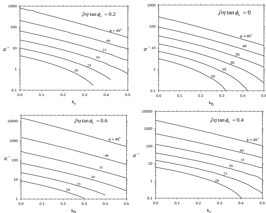
شکل ۵. ضریب ظرفیت باربری N_p به‌ازای مقادیر مختلف \bar{\rho}\eta \tan \phi_w
