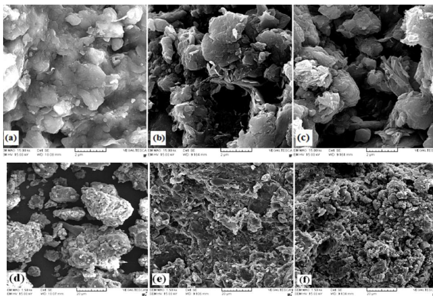
شکل ۸. عکس‌های SEM از نمونه‌های آزمایش شده (a و b) خاک رس (b و e) خاک رس با ۱ درصد آهک (c و f) خاک رس با ۳ درصد آهک
