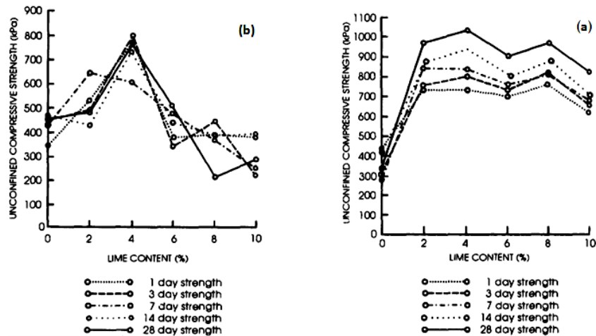
شکل ۱. مقاومت فشاری ساده: (a) کاولینیت، (b) مونتموریلونیت با درصدهای مختلف آهک [۸]
