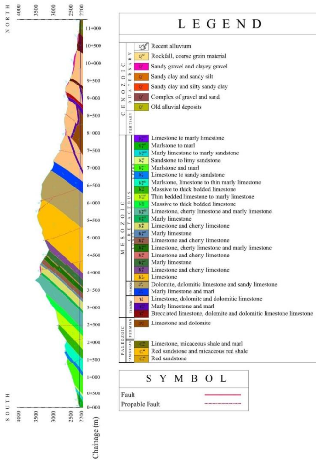
شکل ۲. مقطع زمین شناسی مسیر تونل انتقال آب سبزکوه [۱۷]
