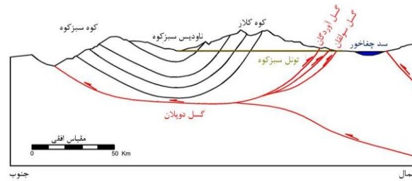
شکل ۳. مقطع ناودیس سبزوکه از سد چغاخور تا محدوده گسل دوپلان [۱۷]
