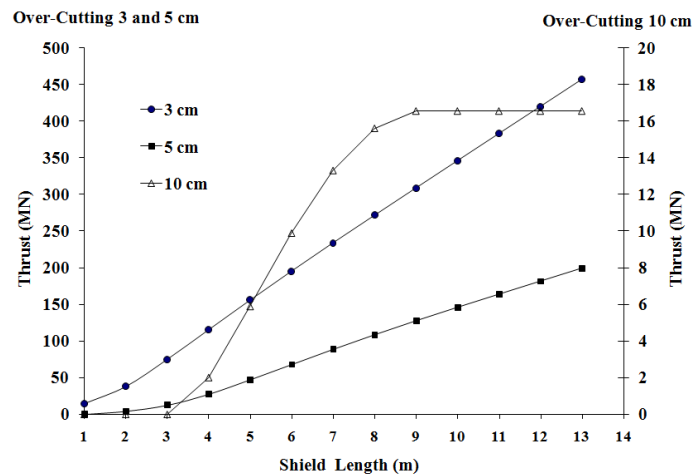
شکل ۳. تغییرات تراست لازم برای غلبه بر اصطکاک بدنه در مقابل طول سپر برای شرایط ژئومکانیکی کمینه در کیلومتر ۳۱۶۰۰-۳۱۶۰۰ و ۲۹۰۳۰-۳۱۶۰۰ و ۳۷۴۹۰-۳۴۹۰۰
