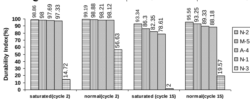
شکل ۹. ارتباط بین شاخص دوام و وارفتگی سیکل دوم ( Id_2 ) و سیکل پانزدهم ( Id_{15} ) برای نمونه‌های مختلف توف که تحت شرایط اشباع و خشک در pH=2.5 آزمایش شده‌اند.
