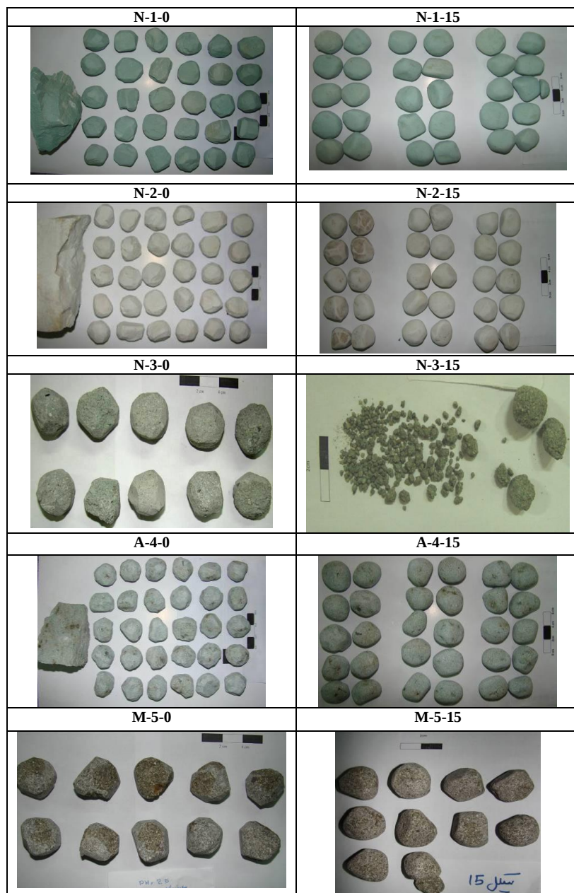
شکل ۶. تغییرات در شکل نمونه و اندازه نمونه‌های دوام بعد از ۱۵ سیکل از انجام آزمون دوام وارفتگی در pH=2.5 ، کدهای بالای هر عکس نشان‌دهنده نوع سنگ (جدول ۱) و تعداد سیکل آزمون دوام است.
