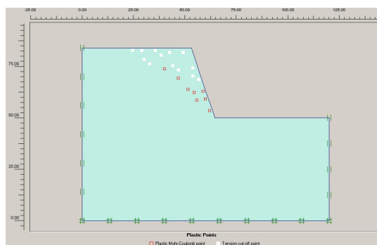
شکل ۵. نقاط پلاستیک شده و تحت کشش در حالت دوبعدی برای ترانسه به ارتفاع ۳۴ متر با شیب ۱ افقی: قائم و مصالح L1-1
