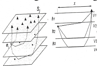
شکل ۴. مسیر موج‌های مستقیم و شکست مرزی حاصل از یک زمین‌لرزه در یک مدل فرضی با لایه‌بندی افقی در زیر شبکه لرزه‌نگاری
