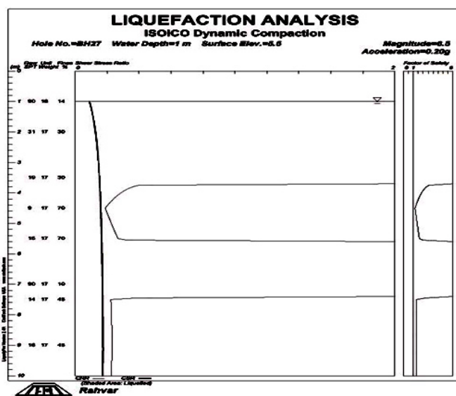
شکل ۱۲. نتیجه تحلیل روان‌گرایی گمانه Z4-BH27 با فرض وقوع زلزله به شتاب g/۲۰ و
