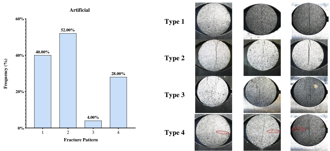
شکل ۹. انواع الگوهای شکست و توزیع آن‌ها در بین ۲۵ نمونه شبه سنگی با فک‌های بارگذاری مختلف Fig. 9. Types of fracture patterns and their distribution among 25 rock-like specimens with different loading jaws
